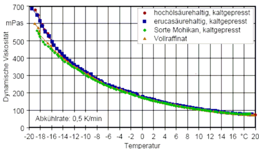
Abbildung 56: Dynamische Viskosität von Rapsöl, gemessen mit einem Rotationsviskosimeter, bei einer Abkühlrate von 0,5 K/min
